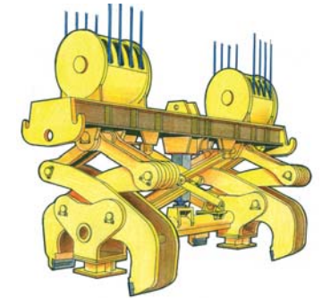
SLAB TRAVERSE GRAB
